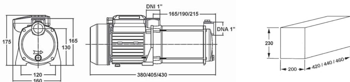
Dimensiones / Dimensions (mm)
